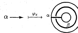
Fig. 10. A map \varphi_\epsilon .
